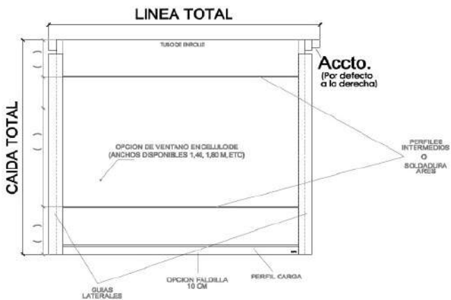
ESQUEMA ORIENTATIVO ARMADO TIPO / FORMATO ( C ) Nº DE PIES ( )
