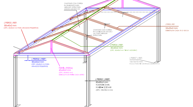
ESQUEMA ORIENTATIVO ARMADO TIPO / FORMATO ( A ) Nº DE PIES: ( )
