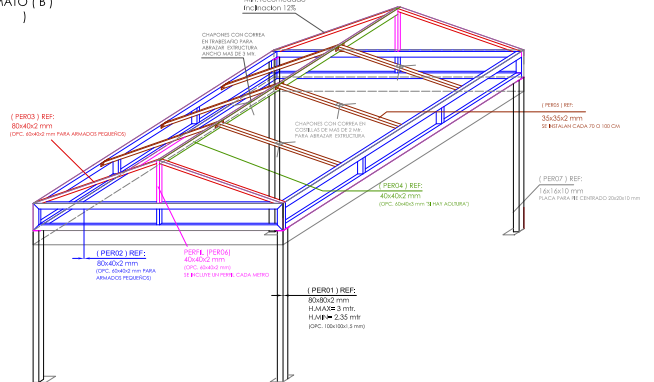
ESQUEMA ORIENTATIVO ARMADO TIPO / FORMATO ( B ) Nº DE PIES: ( )
