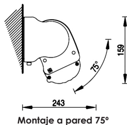
Montaje a pared 75°
