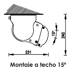
Montaje a techo 15°
