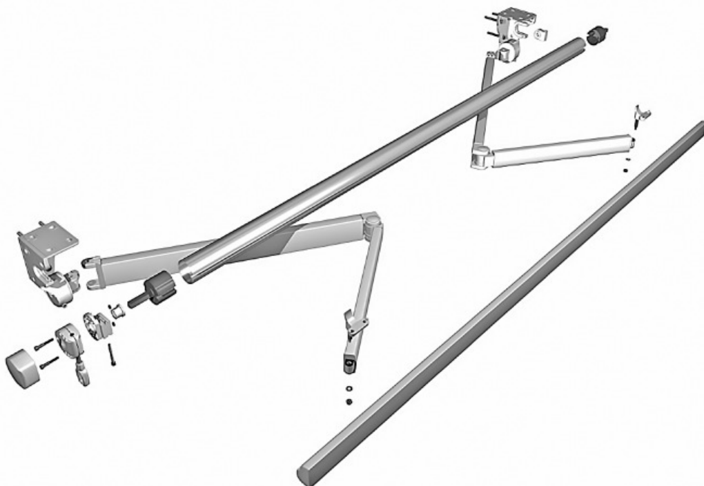
Cambalés despiece
