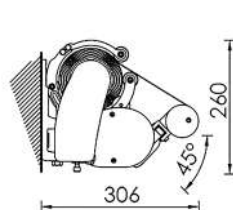
Montaje a pared 45°
