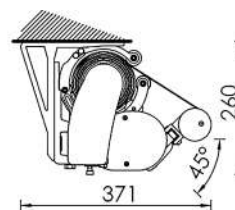
Montaje a techo 45°
