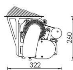
Montaje a techo
