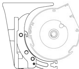
Dimensiones cofre y medidas básicas, soporte pared.
