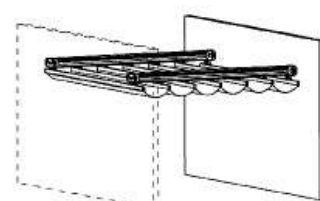
Instalación entre paredes
