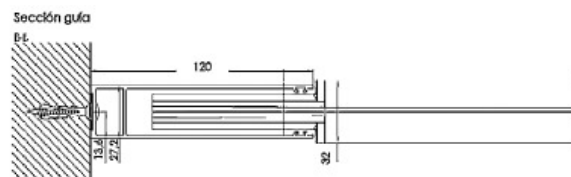
Detalle sección guía
