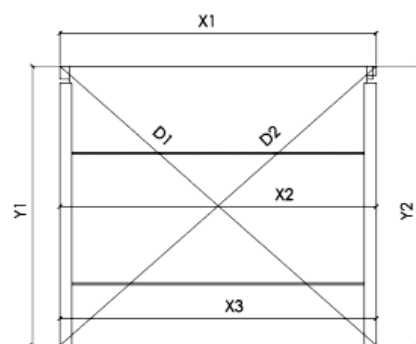
Paraviento medidas
