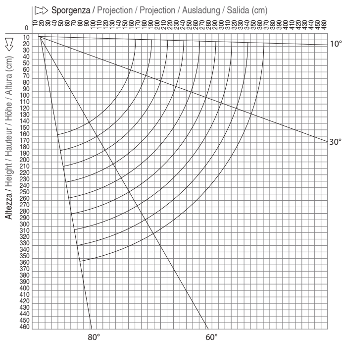
Diagramma di copertura - Installazione a parete
