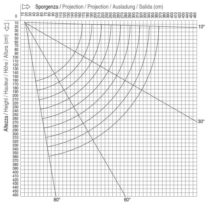
Diagramma di copertura - Installazione a soffitto
