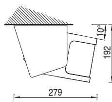
Installazione a soffitto 80°
