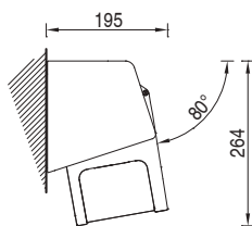
Installazione a parete 80°
