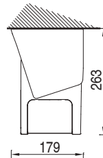
Installazione a soffitto
