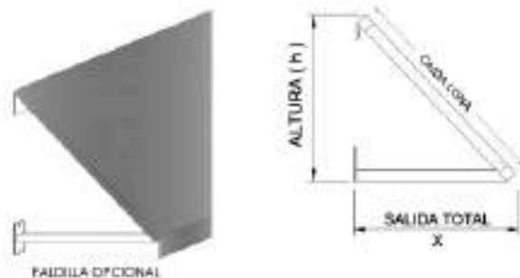
Detalle toldo recto fijo con bastidor
