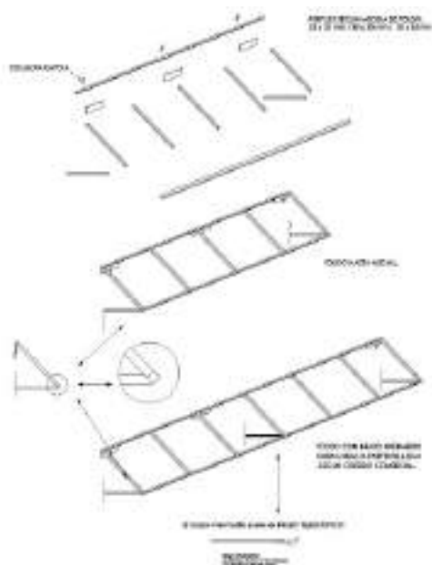
Esquema variables recto fijo con bastidor sin faldilla
