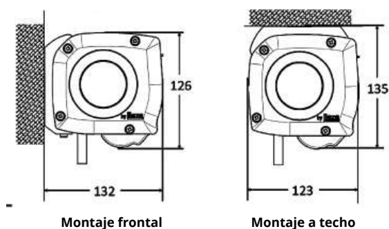
Montaje frontal
