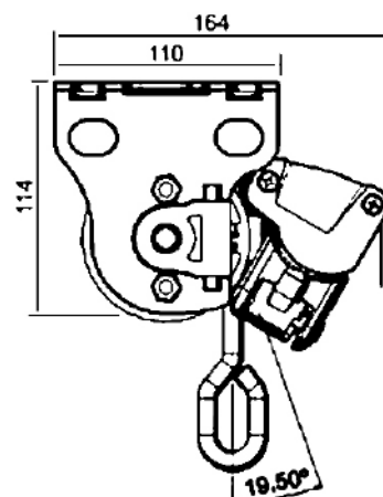
Dimensiones soportes Vertical
